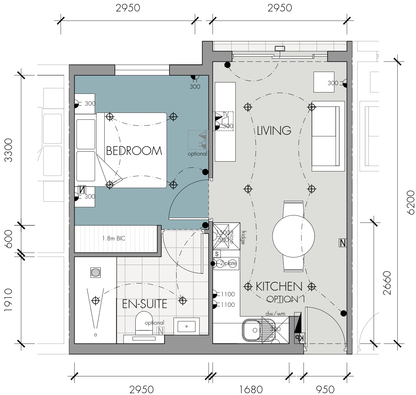
UNIT 3213 SCALE 1 : 50
